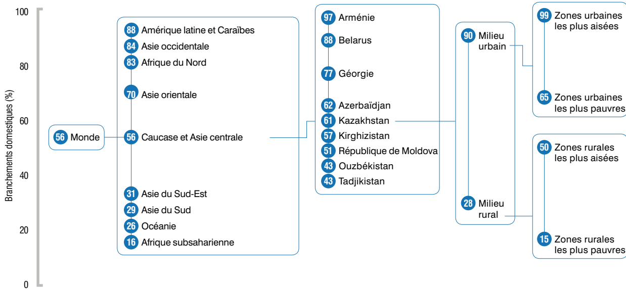
Fig.26 Arbre d'équité pour les branchements domestiques, Kazakhstan, 2012
