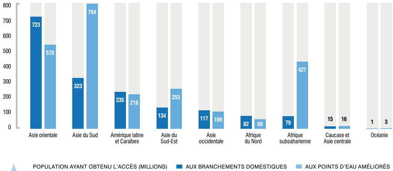
Fig.12 Population ayant obtenu l'accès à des points d'eau améliorés et aux branchements domestiques (1990–2015)
